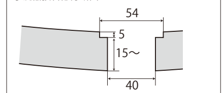
手洗器接合部分断面
